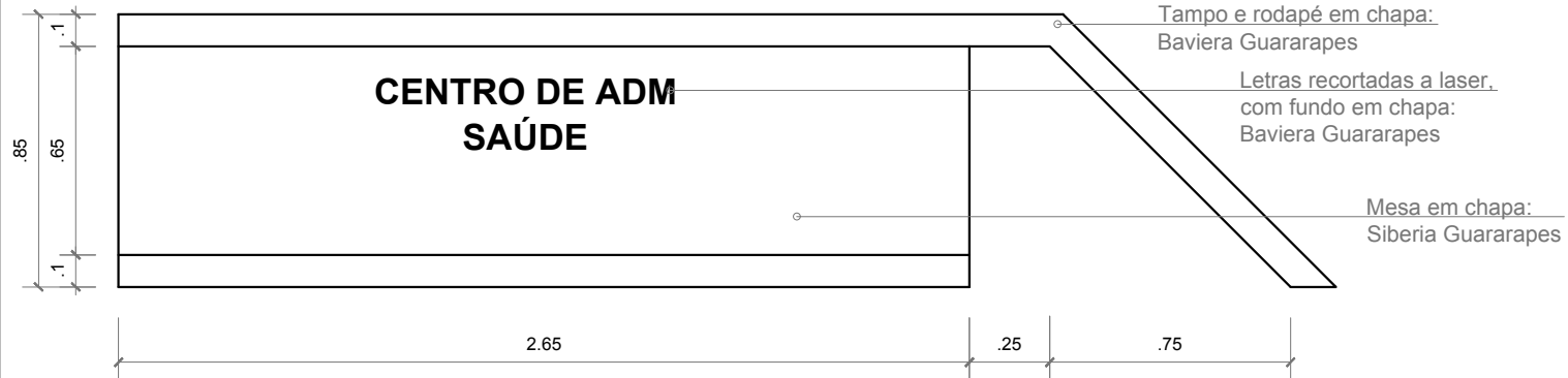
DETALHAMENTO MESA VISTA FRONTAL
