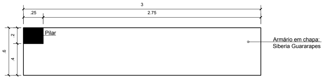
DETALHAMENTO ARMÁRIO VISTA SUPERIOR
