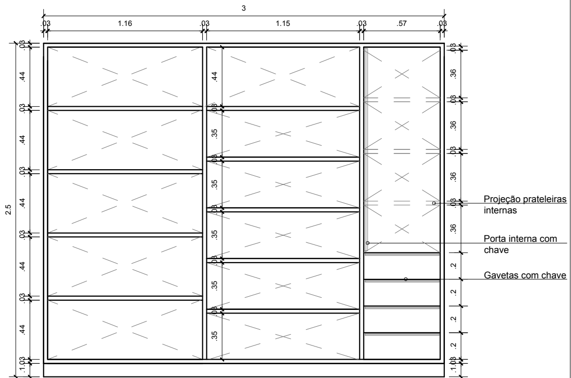
DETALHAMENTO ARMÁRIO VISTA FRONTAL - DIVISÓRIA INTERNA
