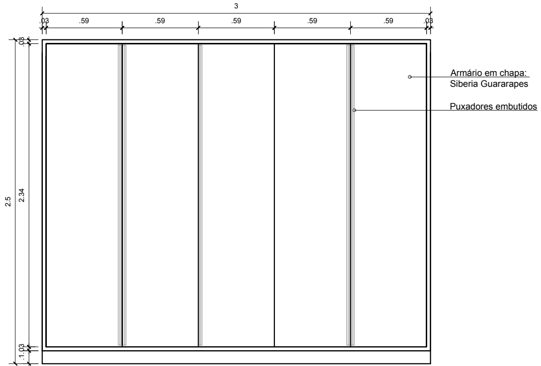
DETALHAMENTO ARMÁRIO VISTA FRONTAL
