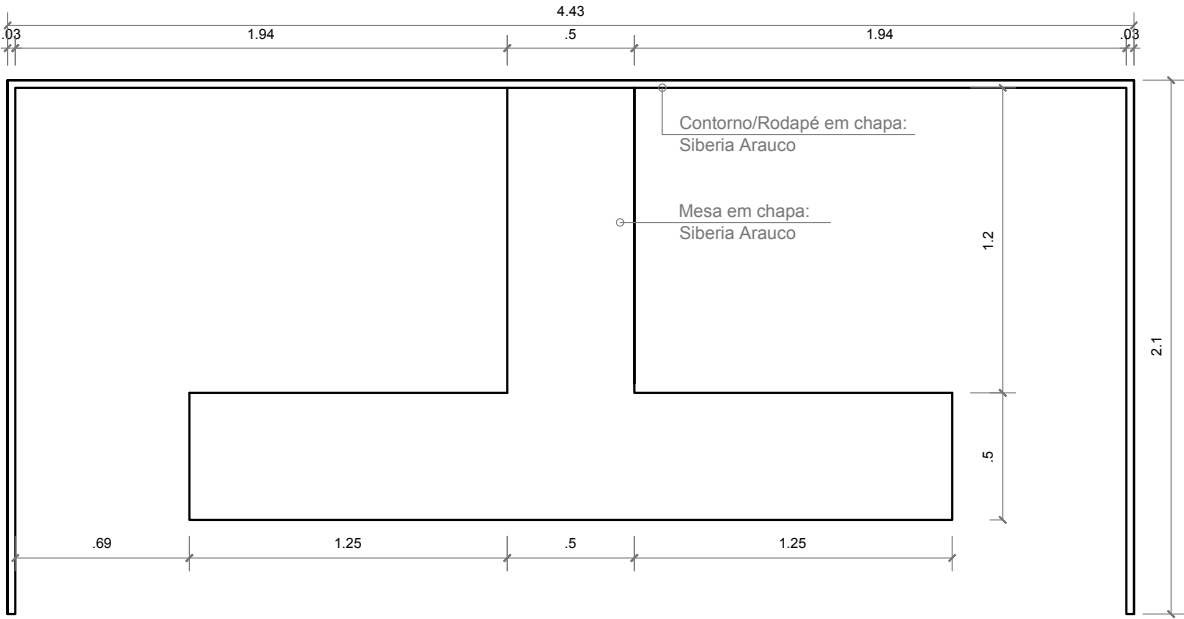
DETALHAMENTO MESA VISTA SUPERIOR
