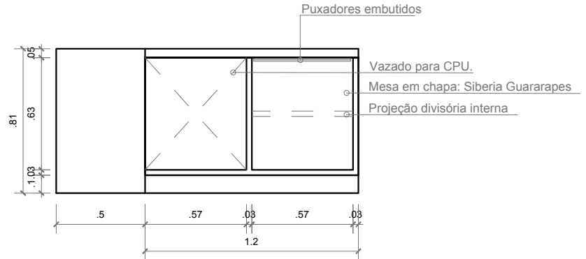
DETALHAMENTO MESA VISTA LATERAL DIREITA
