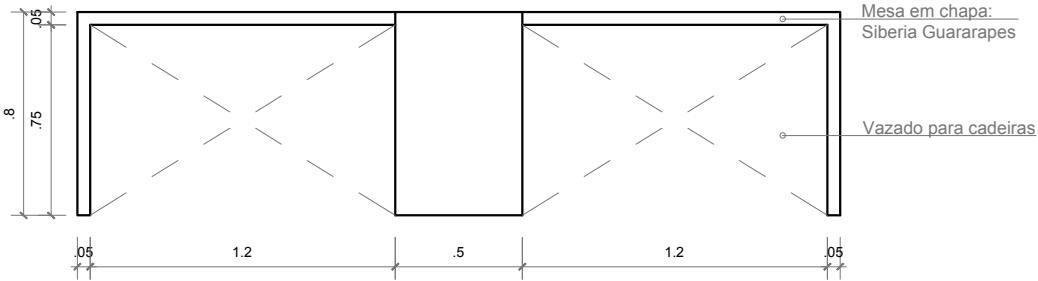
DETALHAMENTO MESA VISTA FRONTAL
