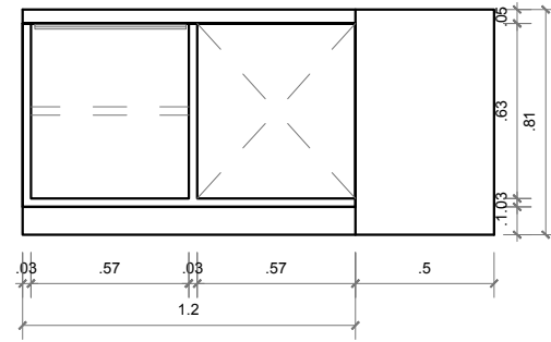
DETALHAMENTO MESA VISTA LATERAL ESQUERDA
