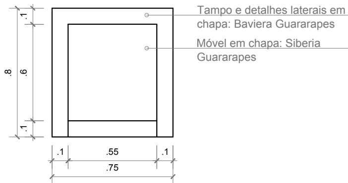
DETALHAMENTO BUFFET VISTA LATERAL
