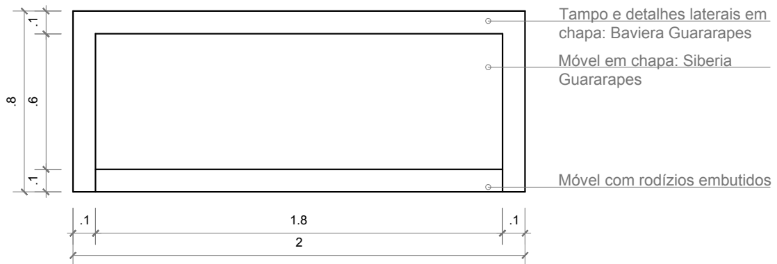
DETALHAMENTO BUFFET VISTA FRONTAL
