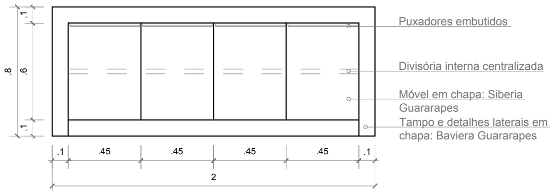
DETALHAMENTO BUFFET VISTA POSTERIOR
