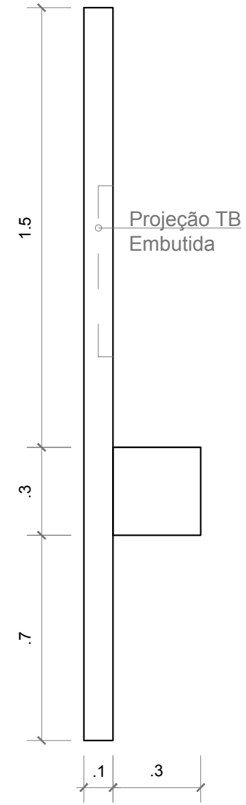
DETALHAMENTO PAINEL TV VISTA LATERAL
